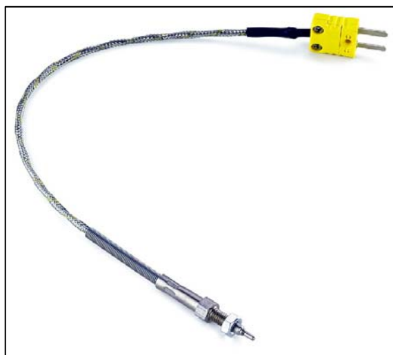
Joonis 5: Väljalaskegaaside temperatuuri mõõtmiseks kasutatav K-Type sensor
